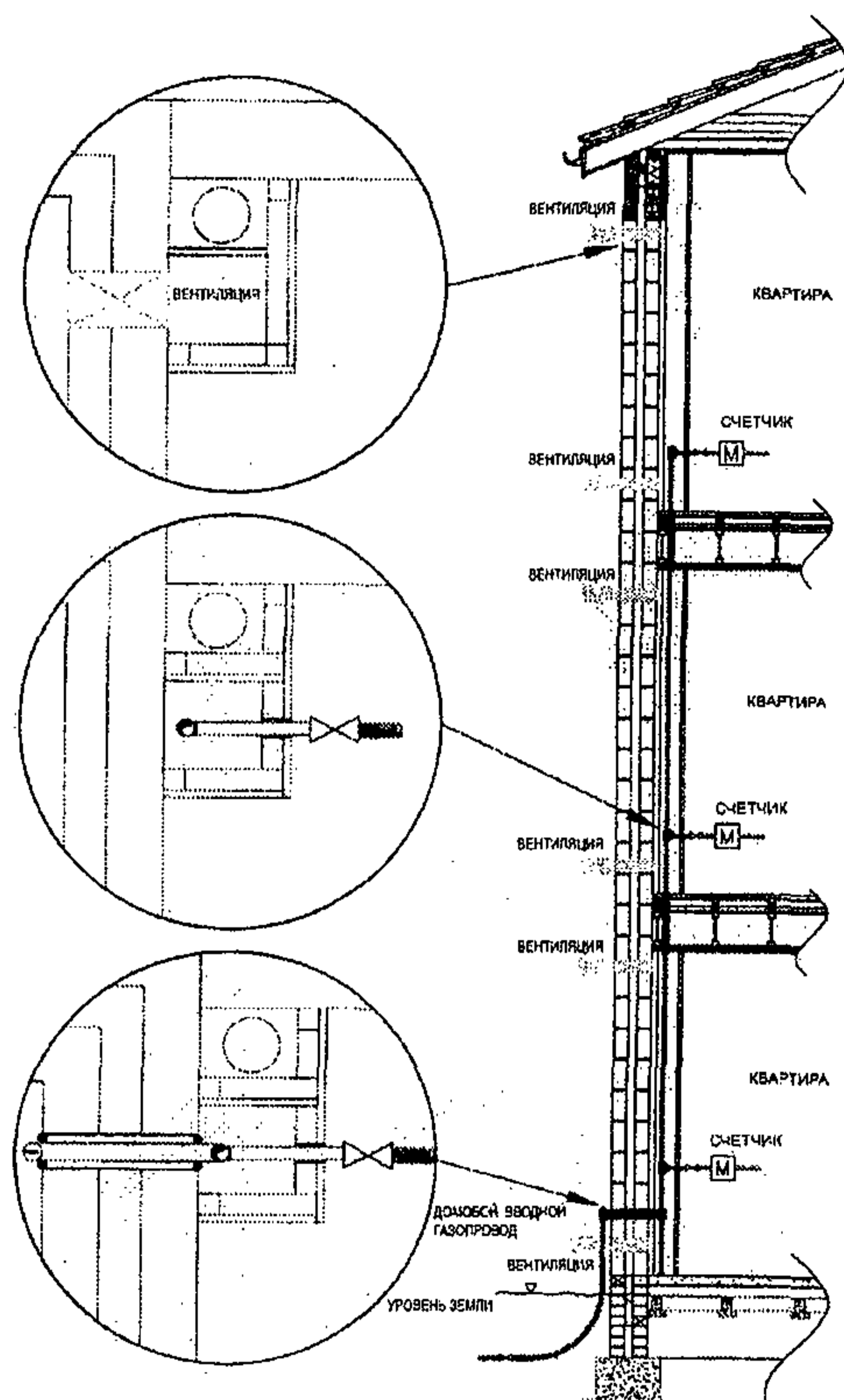
Рисунок Г.1 – Газопровод в вентилируемой штрабе
