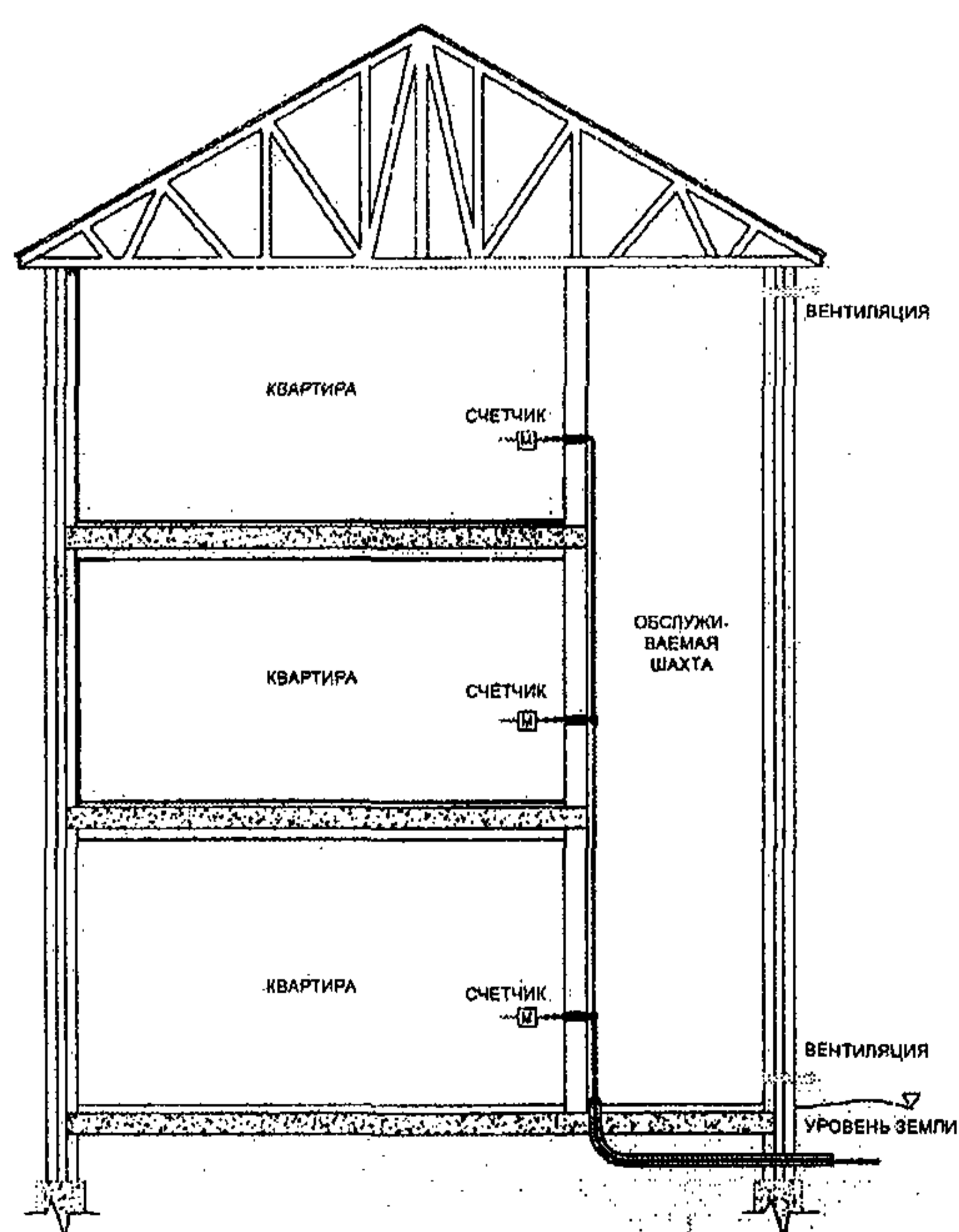
Рисунок Г.2 – Газопровод в вентилируемой шахте
